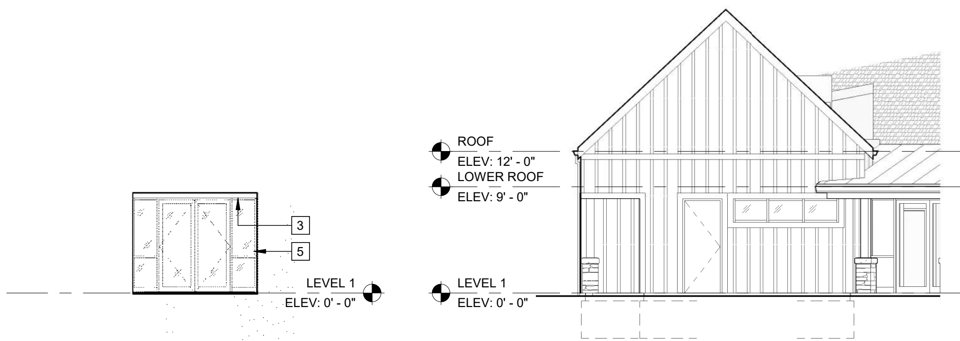
13 NORTH ELEV 5 A-201 Scale: 1/8" = 1'-0"
