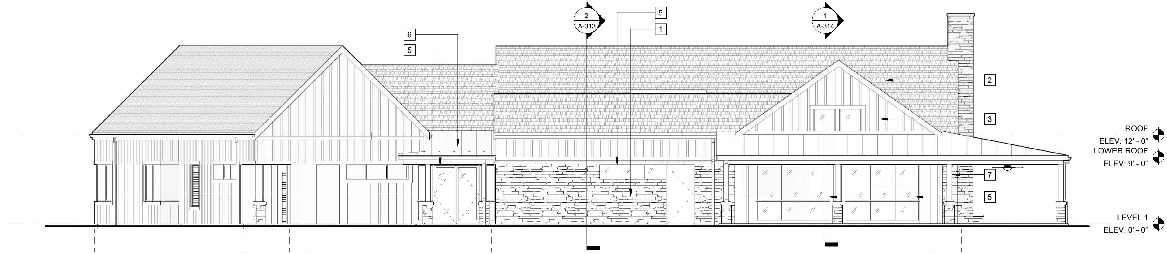
3 NORTH ELEV A-201 Scale: 1/8" = 1'-0"
