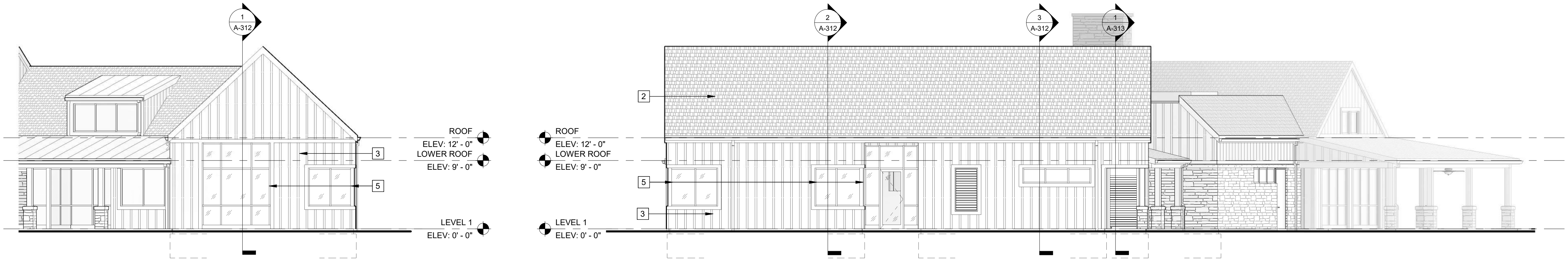
6 SOUTH ELEV 2 A-201 Scale: 1/8" = 1'-0"
