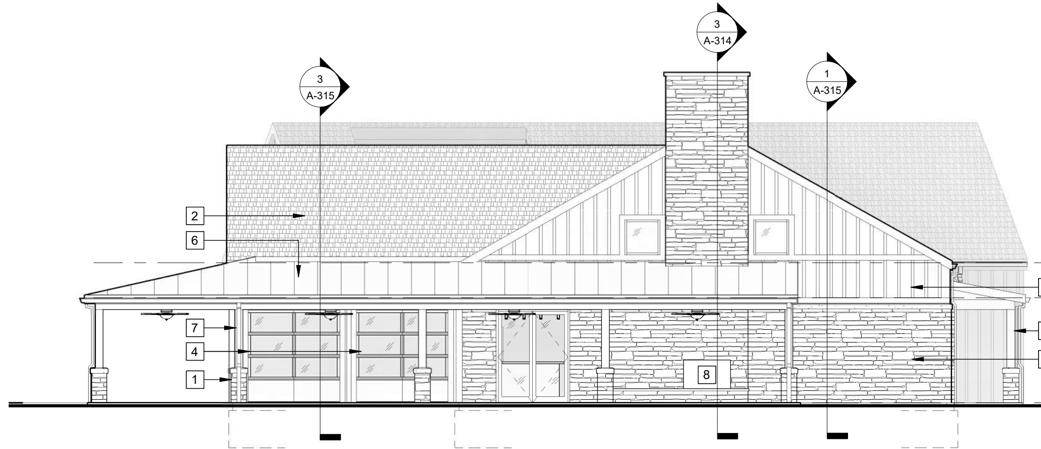
2 WEST ELEV A-201 Scale: 1/8" = 1'-0"
